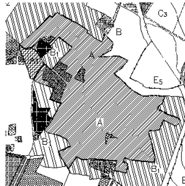
PIANO PARTICOLAREGGIATO
